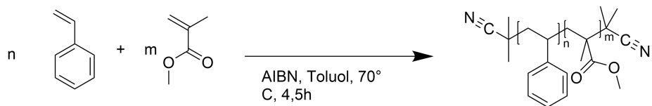
Abb. 15: Reaktionsgleichung zur Synthese von Polystyrol- co -Polymethylmethacrylat über freie radikalische Polymerisation.
